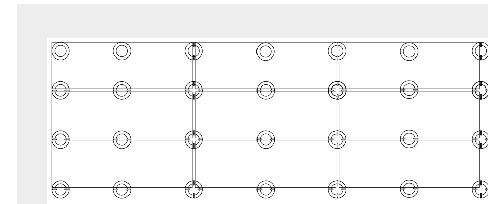
SUPPORTO REGOLA AUTOLIVELLANTE Paving support Verstellbare Stütze Support réglable Soporte regulable Регулируемая опора
